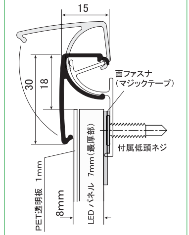
フレーム構造/断面
