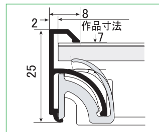
前開き式アルミフレーム（屋内用） 背板：表面コート 紙ダンボール（3mm厚） 透明板：PET樹脂板（0.6mm厚 A0以上は1mm） 付属品：吊り下げヒモ バックスプリング 取扱説明書 サイズ：B0～A4 ※A1以上にスライドロック付属
